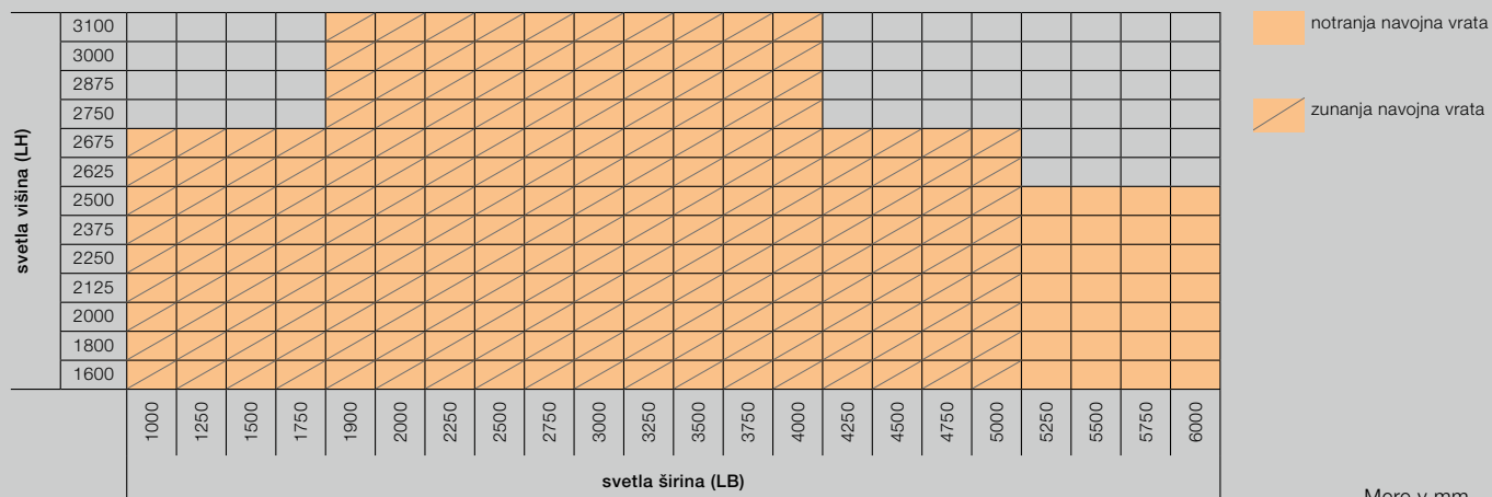
Območje velikosti za notranja in zunanja navojna vrata
